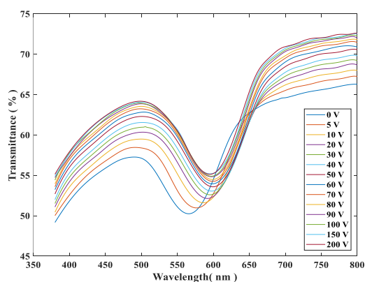
شکل (۳): جابجایی طیفی انعکاس انتخابی براگ برای نمونه ی بلورمایع کلستریک تثبیت شده در پلیمر در حضور میدان الکتریکی
