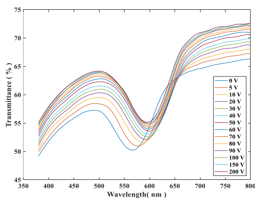
شکل (۳): جابجایی طیفی انعکاس انتخابی براگ برای نمونه ی بلورمایع کستریک تثبیت شده در پلیمر در حضور میدان الکتریکی
