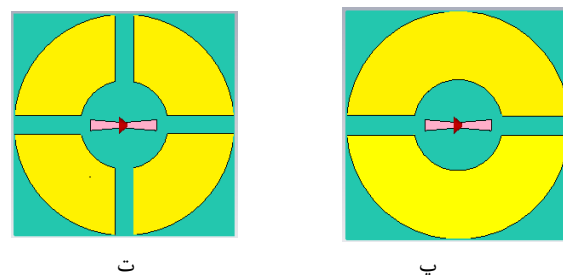
شکل ۱: مراحل مختلف طراحی آنتن پیشنهادی، (الف) دوقطبی فلزی تنها، (ب) آنتن دوقطبی با بارگذاری دو نوار گرافن با پهنای 15\mu m ، (پ) آنتن دوقطبی با بارگذاری دو نوار گرافن با پهنای 75\mu m ، طرح نهایی با چهار نوار ربع دایره گرافنی مجزا با پهنای 75\mu m
