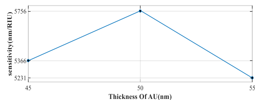
شکل ۴: تغییرات میزان حساسیت سنسور نسبت به تغییر ضخامت لایه طلا از ۴۵ نانومتر به ۵۵ نانومتر با d = 1 \mu\text{m} , \Lambda = 2 \mu\text{m}
