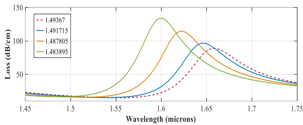
شکل ۵: نمودار تلفات حبس شدگی به ازای ضرایب شکست مختلف روغن با t_{AU} = 50 \text{ nm} , d = 1.1 \mu\text{m} , \Lambda = 2 \mu\text{m}
