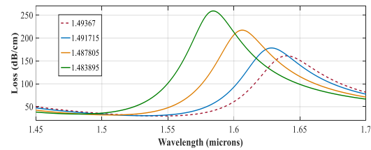
شکل ۳: نمودار تلفات حبس شدگی برحسب طول موج به ازای ضرایب شکست مختلف روغن با t_{AU} = 50 \text{ nm} , d = 1 \mu\text{m} , \Lambda = 2 \mu\text{m}
