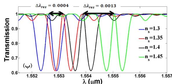
شکل ۳: طیف توان نور عبوری ساختار حسگر فیبر نوری مبتنی بر توری براگ به ازای ضریب شکست‌های مختلف محیط، الف- ساختار بدون انتقال فاز، ب- با انتقال فاز \frac{\pi}{2} در وسط توری.
