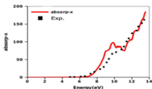
شکل 10: مقایسه نتایج تجربی و محاسباتی ضریب جذب در راستای محور X
