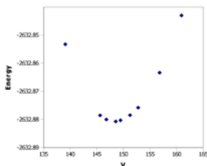
شکل ۲: بهینه سازی انرژی نسبت به حجم
