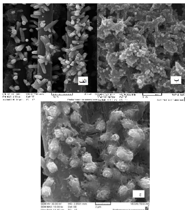
شکل ۴: تصاویر SEM: تصویر الف نانومیله‌های اکسیدروی، تصویر ب نانوسیم‌های پلی‌آنیلین، تصویر ج نانوکامپوزیت اکسیدروی-پلی آنیلین.
