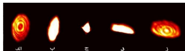
شکل ۴- طرح پراش ثبت شده در فاصله‌ی الف: ۳۱,۵، ب: ۳۶,۵، ج: ۴۰ (کانون)، د: ۴۳,۵، ه: ۴۸,۵ سانتی متری از المان عدسی فرنل.
