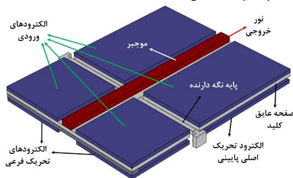
شکل ۱: کلید MEMS پیشنهادی.
