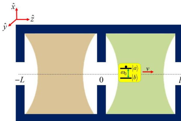
شکل ۱: یک طرحواره کلی از سیستم مورد مطالعه (کیوبیت متحرک با سرعت ثابت v در یک کاواک دوگانه نشانداده)
