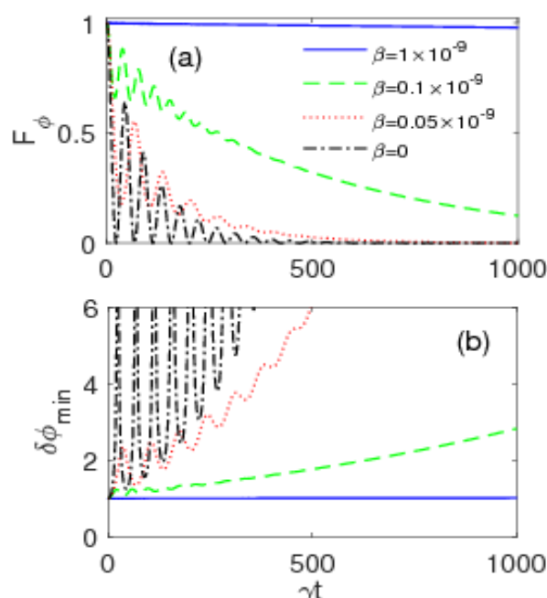
شکل ۲: (a) تحول زمانی F_\phi به ازای سرعت‌های مختلف کیوبیت: (b) تحول زمانی تخمین فاز بهینه \delta\phi_{\min}(t) به ازای سرعت‌های مختلف کیوبیت. مقادیر سایر پارامترها عبارتند از: \alpha = \beta = 1/\sqrt{2} , \omega_0 = 1.53 \times 10^9 \text{ Hz} , \gamma = 33 \text{ Hz} و \Delta = 0 , \lambda = 0.01\gamma
