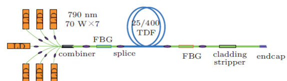
شکل ۱: نمایی از لیزر تمام تاری آلاییده به تولیوم [۴].
