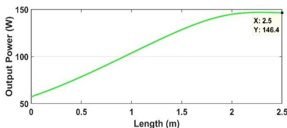
شکل ۳: نمودار شبیه سازی شده توان خروجی لیزر برای طول ۲/۵ متر و بازتابندگی ۱۵ درصد.
