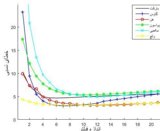
شکل ۲: اثر اندازه فیلتر میان گذر بر روی دقت اندازه گیری مورفولوژی نمونه مکعبی (نمودار تغییرات خطای نسبی بر حسب اندازه ی فیلتر (تعداد پیکسل) برای نمونه کروی)
