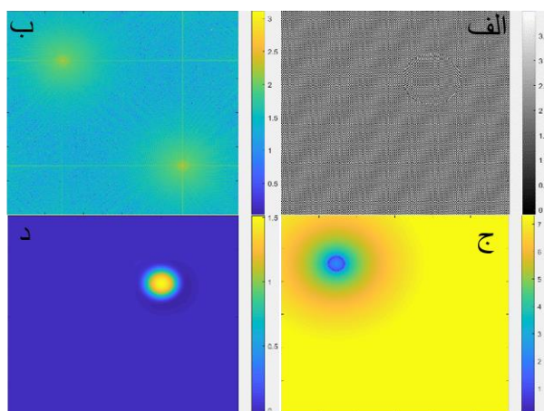
شکل ۱: بازسازی تصویر یک مهره به کمک الگوریتم استخراج فاز ((الف) تصویر شدت مهره در داخل طرح تداخلی (ب) تبدیل فوری ی طرح شدت در فضای فرکانس (ج) تصویر در فضای فرکانس تحت تاثیر یک فیلتر مناسب (د) نتیجه بازسازی تصویر پس از الگوریتم واپیچی ) این فیلترها، با تغییر اندازه ی آن فیلتر بهینه را مشخص نمودیم.
