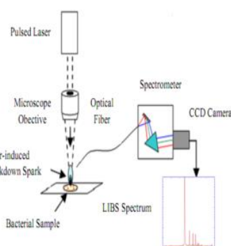
شکل ۱: طرحواره نوعی از چیدمان آزمایش [۵].
