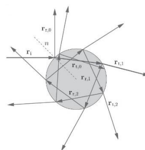
شکل ۲- بازتاب‌های متوالی تک پرتو داخل کره دی‌الکتریک
