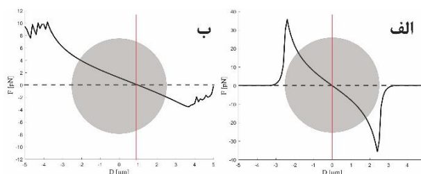
شکل ۳- الف) نیروی وارد بر ذره در فواصل مختلف از کانون در راستای x در z = 5.1 \mu m ب) نیروی وارد بر ذره در فواصل مختلف از کانون در راستای z و در x = 0 .
