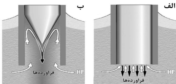
شکل ۲ - نحوه تشکیل مخروط توسط جریان همرفتی اسید خورنده و فرآورده‌های واکنش الف ب
