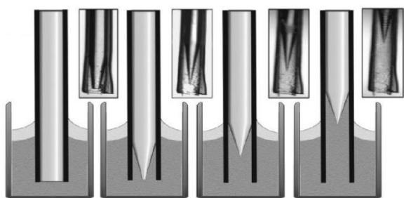
شکل ۱ - مراحل تشکیل مخروط داخل روکش فیبر الف ب ج د
