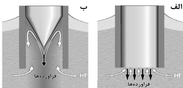
شکل ۲ - نحوه تشکیل مخروط توسط جریان همرفتی اسید خورنده و فرآورده‌های واکنش
