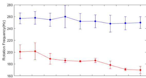
شکل ۴: نمودار تغییرات سرعت چرخش ذره اول با دور شدن ذره دوم بر حسب فاصله بین دو ذره را نشان می‌دهد. داده‌های آبی و قرمز به ترتیب مربوط به قطبش موازی و عمود بر خط واصل دو ذره است.
