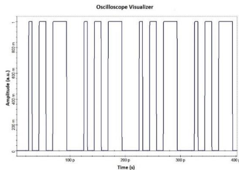
شکل ۲: سیگنال ورودی ۱ (۰۱۰۰۱۱۰۰۱۱۱۱۰۰۰۰)
