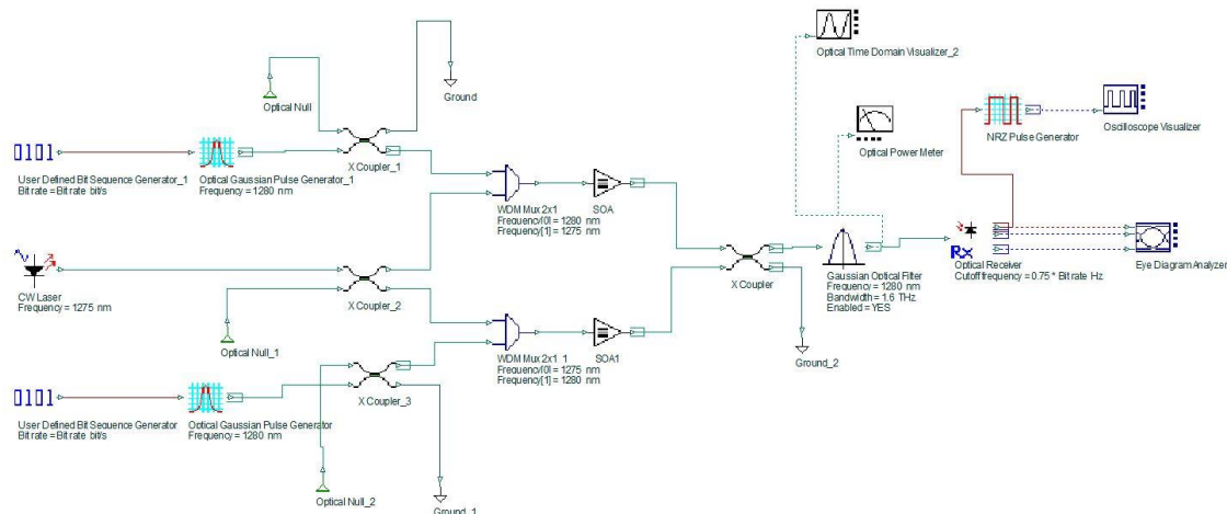
شکل ۱: نمای کلی گیت XOR با استفاده از تقویت کننده نوری نیمه هادی و تداخل سنج ماخ زندر.
