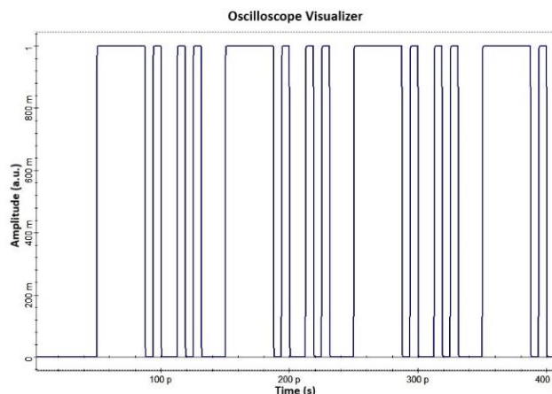
شکل ۴: سیگنال خروجی گیت XOR.
