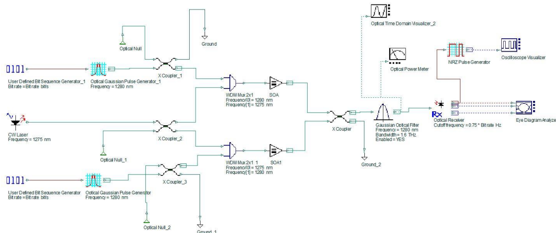
شکل ۱: نمای یک گیت XOR با استفاده از تقویت کننده نوری نیمه هادی و تداخل سنج ماخ زندر.
