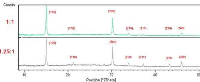
شکل ۲: طیف پراش اشعه ایکس از لایه نازک پروسکایت برای دو نسبت ۱:۱ و ۱/۲۵:۱ پیش ماده ها
