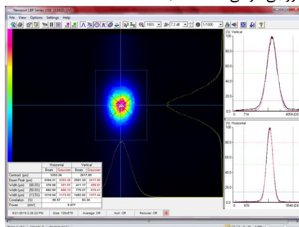
شکل ۶: پروفایل فضایی لیزر پیکوثانیه قفل شده مدی انفعالی.
