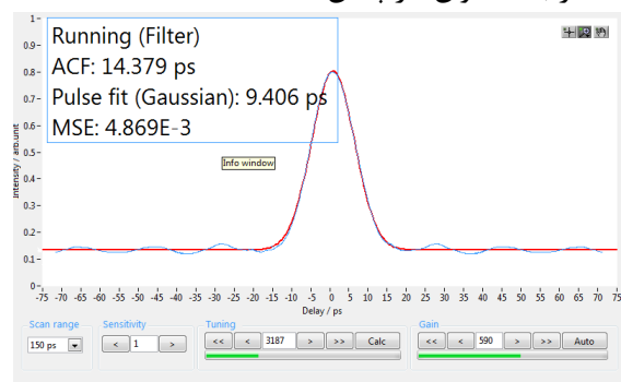
شکل ۵: پروفایل زمانی پالس های قفل شده مدی.
