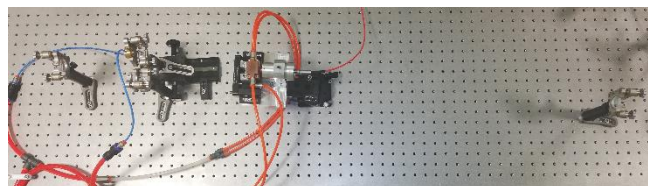
شکل ۳: طرحواره و چیدمان آزمایشگاهی لایزر Nd:YVO4 قفل شده مدی انفعالی.
