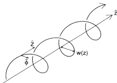
شکل ۱) منحنی مارپیچی بردار پوینتینگ برای باریکه‌ی لاگر-گوسی [۸].
