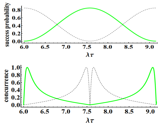
نمودار ۳: نمودار تلاقی و احتمال موفقیت بر حسب \lambda\tau برای \hbar = 1 بر اساس رابطه‌های (۱۷) و (۱۸). در نمودارها C^i(\tau) ، P_{1,8}^i(\tau) با خط پیوسته و C^{i'}(\tau) ، P_{1,8}^{i'}(\tau) با خط چین نمایش داده شده‌اند.
