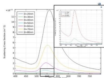
شکل ۴ سطح مقطع پراکندگی برای نانو ذرات با ابعاد ۲۰، ۳۰، ۴۰، ۵۰، ۶۰، ۷۰، ۸۰ نانومتر
