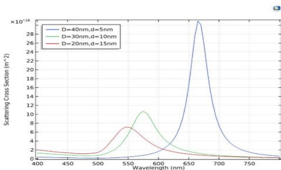
شکل ۷ سطح مقطع پراکندگی نانوذرات با اندازه ۵۰ نانومتر با سایز هسته و پوسته ۵/۴۰، ۱۰/۳۰، ۱۵/۲۰ نانومتر
