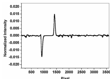
شکل ۴. مشتق سیگنال جسم پس از اعمال فیلتر
