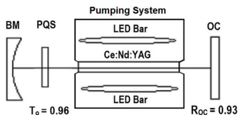
شکل ۳: تشدیدگر نوری به همراه سامانه دمش و سوئیچ نوری انفعالی PQS برای انجام فرایند سوئیچ Q .
