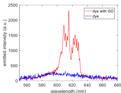
شکل ۷: مقایسه‌ی طیف‌های تابشی نمونه‌های رنگ تنها و محلول رنگ و گرافن اکساید در چگالی انرژی دمش 0.20 \text{ J/cm}^2 .
