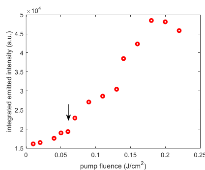
شکل ۶: انتگرال شدت بر حسب چگالی انرژی دمش.
