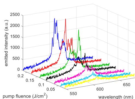
شکل ۴: تغییر طیف گسیل بر حسب طول موج با افزایش چگالی انرژی دمش.
