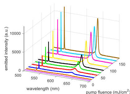
شکل ۳: تغییر طیف گسیل بر حسب طول موج با افزایش چگالی انرژی دمش، متناظر با نمونه‌ی S1 هنگامی که موقعیت دلخواه P1 پمپ شود.
