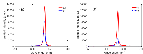
شکل ۵: طیف گسیل بر حسب طول موج برای نمونه‌های S1 و S2 در موقعیت‌های دمش مختلف: الف) P1 و ب) P2.
