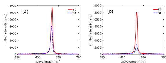
شکل ۵: طیف گسیل بر حسب طول موج برای نمونه‌های S1 و S2 در موقعیت‌های دمش مختلف: الف) P1 و ب) P2.
