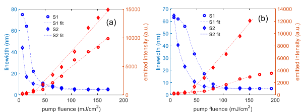
شکل ۶: مقایسه‌ی رفتار آستانه برای نمونه‌های S1 و S2 مربوط به موقعیت‌های دمش مختلف: الف) P1 و ب) P2.
