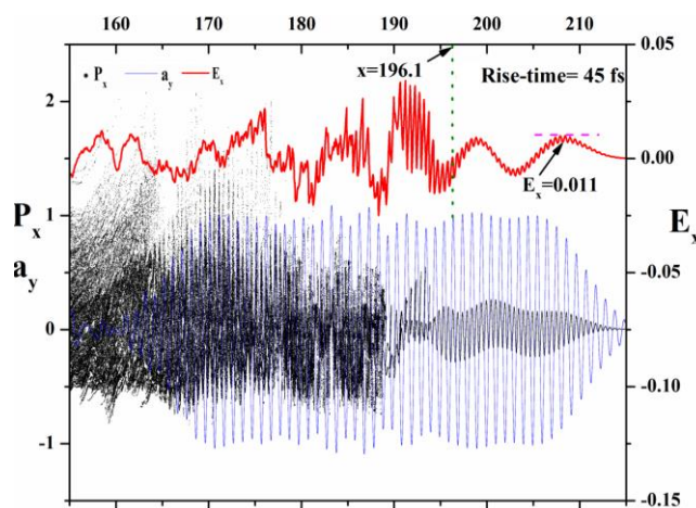
شکل ۲: نمودار فضای فاز، پتانسیل برداری، میدان الکتروستاتیکی، و چگالی الکترون ها برای پالس با زمان خیزش ۴۵ فمتو ثانیه در زمان ۴۸۰ فمتو ثانیه
