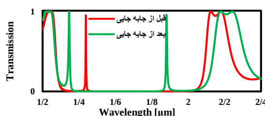
شکل ۲: طیف عبور فیلتر فابری-پرو قبل و بعد از جابه جایی جرم معلق
