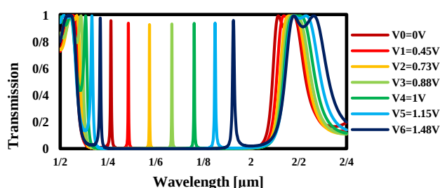
شکل ۵: طیف های عبوری به ازاء ولتاژهای مختلف
