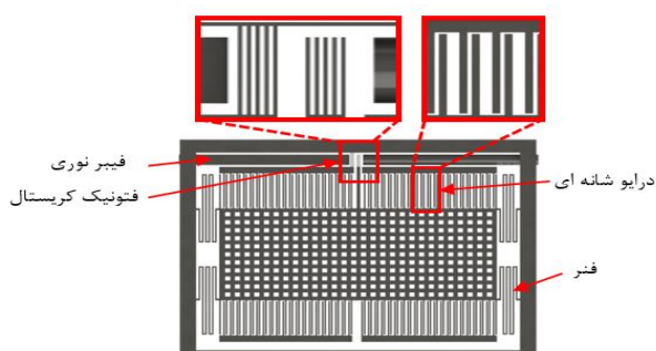
شکل ۱: ساختار محرک MOEMS فیلتر فابری پرو
