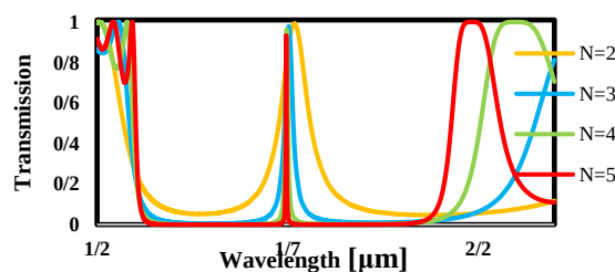
شکل ۴: مقایسه طیف های عبور با افزایش N تعداد لایه ها.
