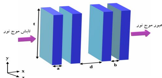
شکل ۳: شماتیک ساختار فوتونیک کریستال یک بعدی. ارتفاع آینه های DBR برابر 10μm، ضخامت هر لایه، a و فاصله بین شان، b هر دو برابر 0.25μm و d فاصله ی DBR ها از هم.
