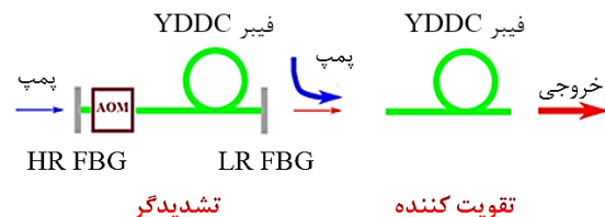
شکل ۱: طرح لیزر فیبری سوئیچ Q؛ در شکل: AOM: المان آکوستو اپتیک، FBG: تار نوری براگ
