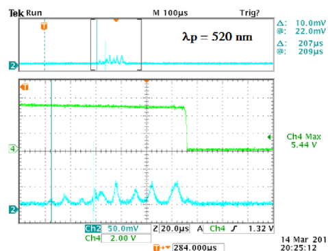
شکل ۵: رفتار زمانی میخه های لیزر (آبی) برای LED با گسیل در ۵۲۰ نانومتر. بخش انتهایی پالس جریان (سبز) با دامنه ۵۴/۴ آمپر.
