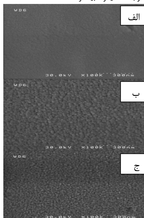
شکل ۵: تصاویر SEM (الف) بدون بازپخت (ب) بازپخت ۴۵۰ درجه سانتیگراد (ج) بازپخت ۵۰۰ درجه سانتیگراد.
