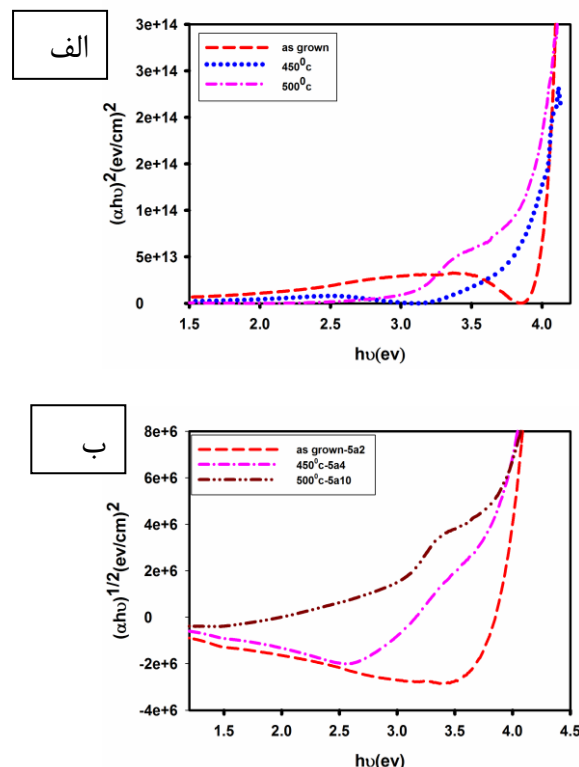
شکل ۴: نمودار الف) (\alpha h\nu)^2 گاف مستقیم
