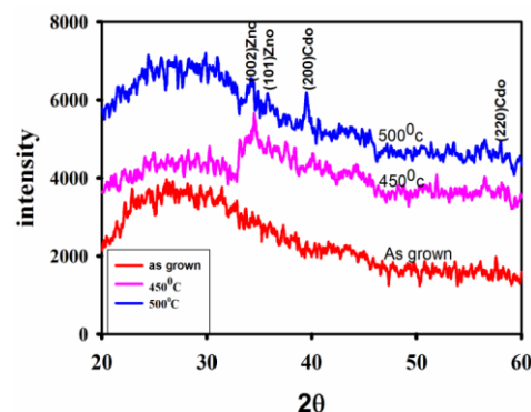
شکل ۴: طیف‌های XRD نمونه‌های بدون بازپخت و بازپخت‌شده در دماهای ۴۵۰ و ۵۰۰ درجه سانتیگراد.
