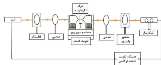
شکل ۱: طرحواره‌ی از چیدمان فارادی.
