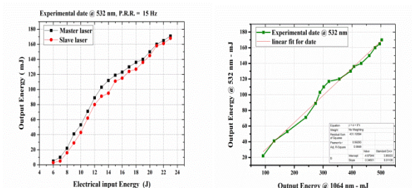
شکل ۸: نتایج انرژی خروجی لیزر در طول موج ۵۳۲ نانومتر بر حسب انرژی ورودی الکتریکی (سمت چپ)، انرژی خروجی در طول موج ۵۳۲ نانومتر بر حسب انرژی خروجی در طول موج ۱۰۶۴ نانومتر (سمت راست)
