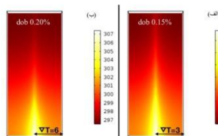
شکل ۵: پروفایل دمایی کریستال تیتانیوم سفایر برای ۱ ثانیه تابش ۵ وات در محیط آزاد. الف: آلایش ۰/۱۵٪ و ب: آلایش ۰/۲۰٪
