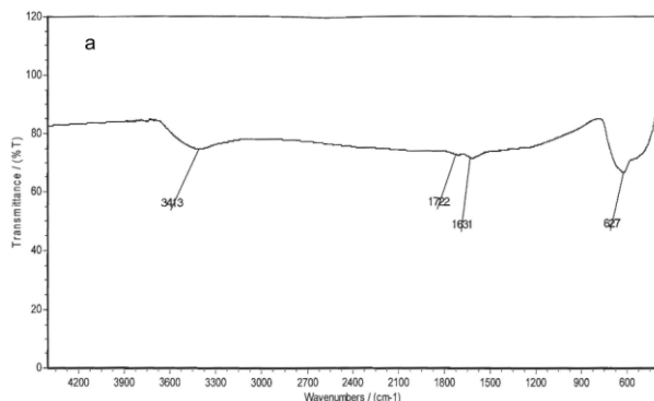
شکل ۵. طیف FT-IR نانوذرات \text{SnO}_2 آلاینده با بورن (۳٪)
