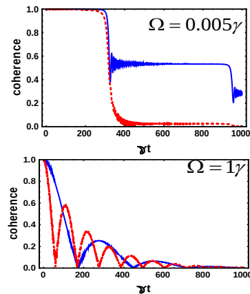
شکل ۲: همدوسی بر حسب \mathcal{H} به‌ازای \delta = 5\gamma ، \lambda = 0.01\gamma برای مقادیر \Omega = 0.005\gamma و \Omega = 1\gamma رسم شده است. خطوط پیوسته آبی و نقطه‌چین قرمز به ترتیب متناظر با گذارهای دو و چهارفوتونی است.
