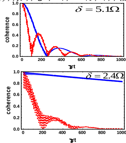
شکل ۳: همدوسی بر حسب \mathcal{H} به‌ازای \Omega = 0.5\gamma ، \lambda = 0.01\gamma برای مقادیر \delta = 5.1\Omega و \delta = 2.4\Omega رسم شده است. خطوط پیوسته آبی و نقطه‌چین قرمز به ترتیب متناظر با گذارهای دو و چهارفوتونی است.
