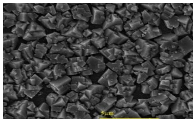
شکل ۴: تصویر SEM مربوط به دمای غوطه‌وری ۲۵°C
