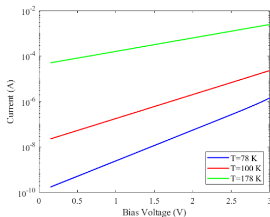
شکل ۳: جریان تاریکی آشکارسازهای Ge/Si
