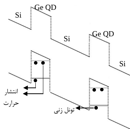
شکل ۲: تصویر شماتیکی از ساختار نواری Ge/Si
