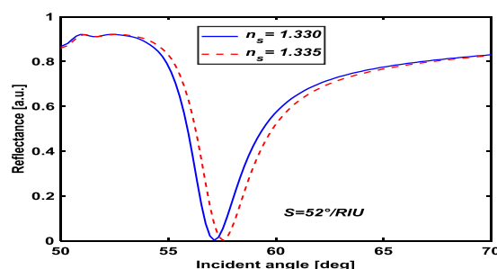
شکل ۲: منحنی تشدید پلاسمون‌های سطحی برای یک زیست حسگر معمولی با فلز طلا به ضخامت ۵۰ نانومتر (بدون لایه گرافنی)
