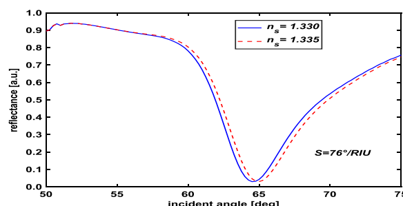
شکل ۳: منحنی تشدید پلاسمون‌های سطحی زیست حسگر پیشنهادی. ضخامت طلا و آلومینیوم اکساید و گرافن به ترتیب برابر است با ۵۰ و ۲۰ و ۰.۳۴ نانومتر.
