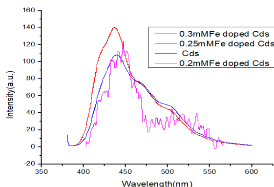
شکل ۶: طیف فوتولومینسانس بر حسب طول موج
