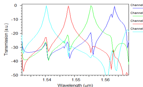
شکل ۶: نمودار هم‌شنوایی در دی‌مالتی‌پلکسر چهار کاناله.
