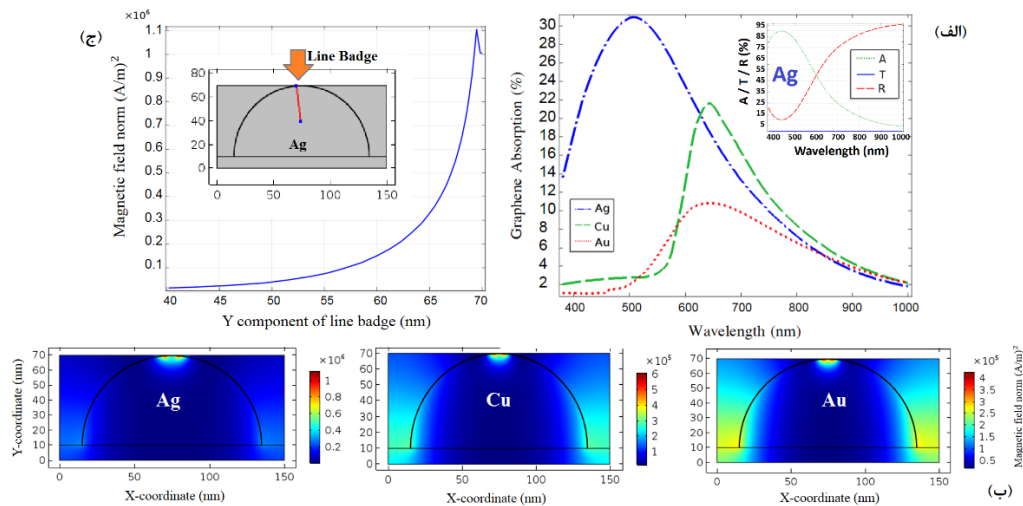
شکل ۲. (الف) مقایسه طیف جذبی گرافن در حضور نقره، مس و طلا. (ب) مقایسه طرح دو بعدی توزیع شدت میدان مغناطیسی بر حسب فاصله از محور xها در حضور سه فلز نقره، مس و طلا و (ج) طرح اندازه شدت میدان مغناطیسی بر حسب مؤلفه y خط نشان در حضور نقره.
