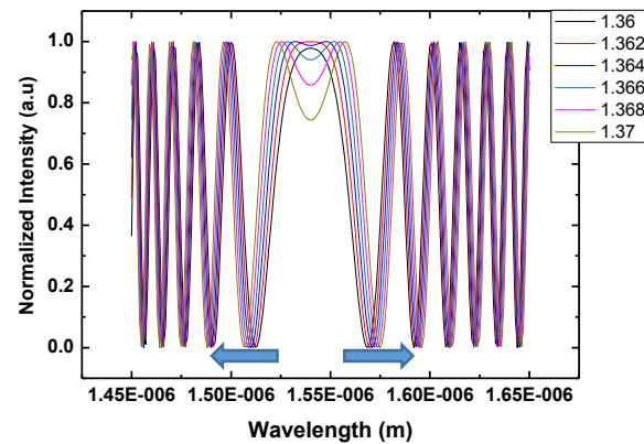
شکل ۲: نمودار جابجایی طول موجی طیف تداخلی با تغییر ضریب شکست محیط خارجی در بازه ی ۱,۳۶ تا ۱,۳۷
