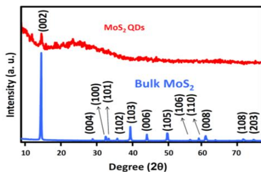
شکل ۱: الگوی پراش پرتو ایکس نقاط کوانتومی دی سولفید مولیبدن ساخته شده در مقایسه با حالت توده ای آن
