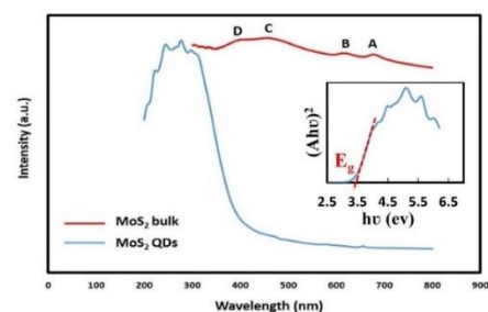
شکل ۲: طیف جذب نقاط کوانتومی ساخته شده دی سولفید مولیبدن در مقایسه با حالت توده ای آن و محاسبه گاف انرژی نمونه نقاط کوانتومی ساخته شده به روش تاک پلات
