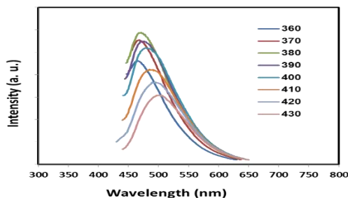
شکل ۳: طیف فوتولومینسانس نقاط کوانتومی ساخته شده دی سولفید مولیبدن در تحریک های مختلف
