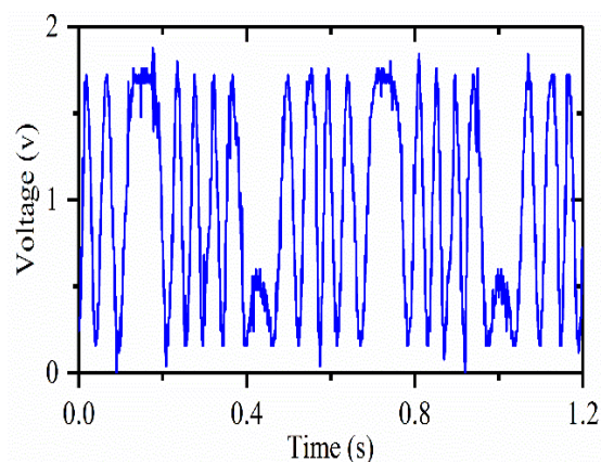
شکل ۴: پاسخ حسگر به نیرویی با دامنه جابجایی ۱/۱۲ mm به مرکز میلگرد
