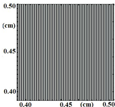
شکل ۴: تصویر هولوگرافی تشکیل شده در 1\text{ mm} انتهای بالایی فیلم برای شیء ۲ و لیزر.
