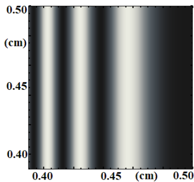
شکل ۳: هولوگرام 1\text{ mm} بالای فیلم در حضور شیء ۱ و لیزر.
