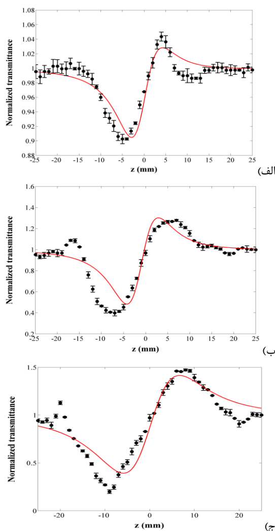
شکل ۳. داده های رویش Z روزنه بسته (نقاط) و برازش (خط قرمز) برای نمونه های الف) \text{TiO}_2 2% PS، ب) \text{TiO}_2 4% PS و ج) \text{TiO}_2 6% PS.
