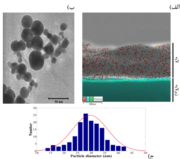
شکل ۲. الف) تصویر SEM سطح مقطعی لایه نانوکامپوزیت PS-6% TiO2. ب) تصویر میکروسکوپ الکترون عبوری نانوذرات و ج) توزیع اندازه نانوذرات.
