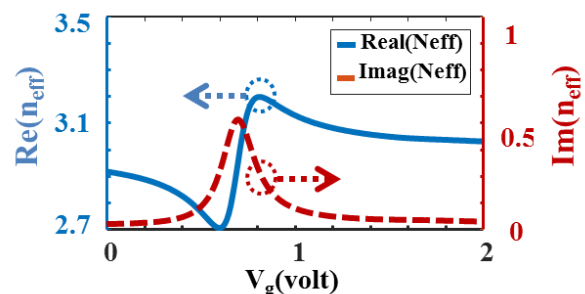
شکل ۲: تغییرات ضریب شکست مد بر حسب ولتاژ اعمالی
