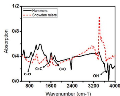
شکل ۳: نتیجه آنالیز طیف‌سنجی تبدیل فوریه مادون قرمز اکسیدگرافن تهیه شده به روش اسنودن مایر و روش هامرز اصلاح شده
