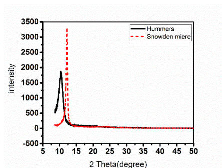
شکل ۱: الگوی پراش اشعه ایکس اکسیدگرافن تهیه شده به روش اصلاح شده هامرز و اسنودن مایر
